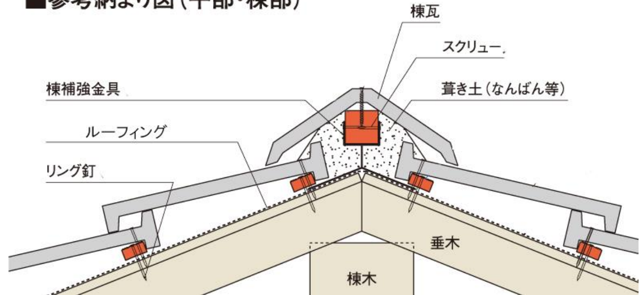
■参考納まり図(平部・棟部)
